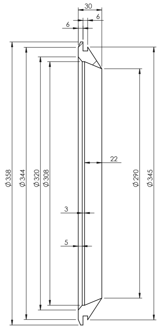
SEZIONE A-A
